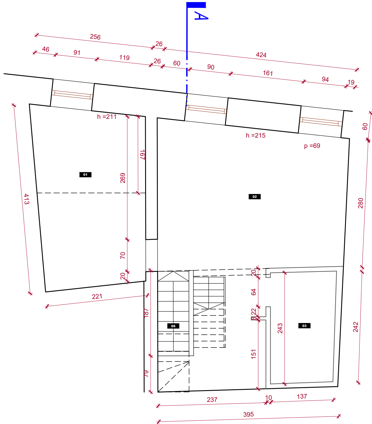
tlocrt galerija M 1:50
